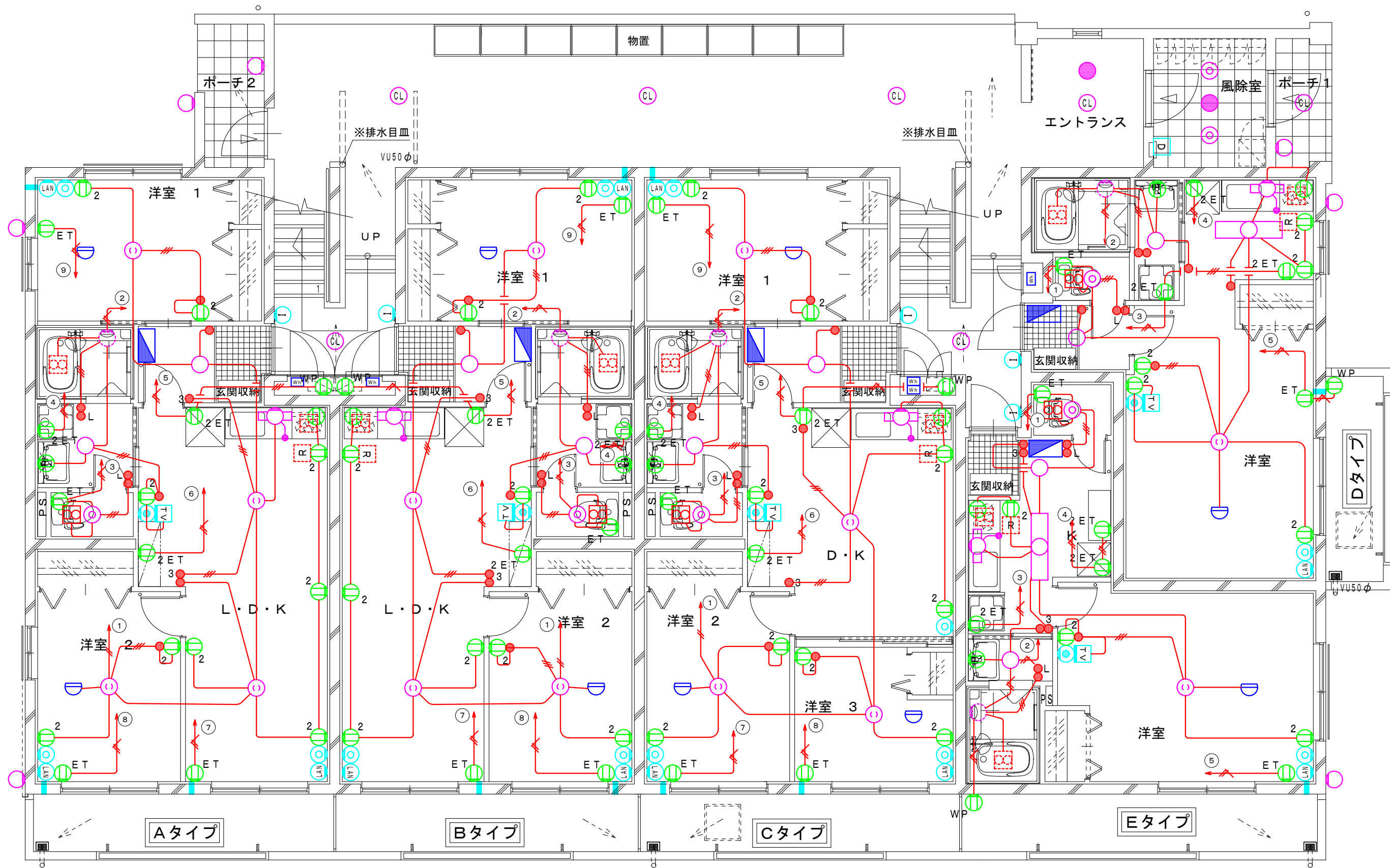
【配線図例】
